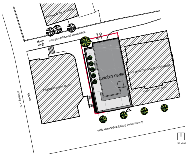
Situácia
