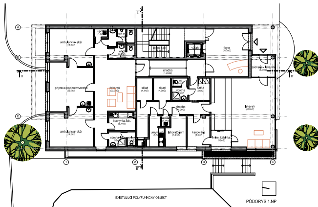
Pôdorys 1. NP
